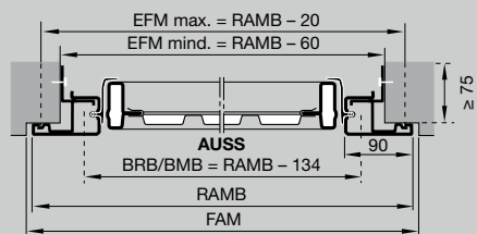
Montage par pinces (profondeur jour min. 50 mm, max. 100 mm)
