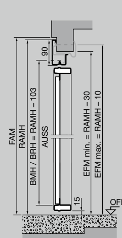
Montage par pinces sans seuil
