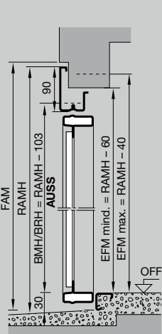
Montage par chevilles avec seuil
