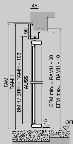
Montage par chevilles sans seuil
