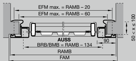
Montage par pinces (profondeur jour min. 50 mm, max. 100 mm)
